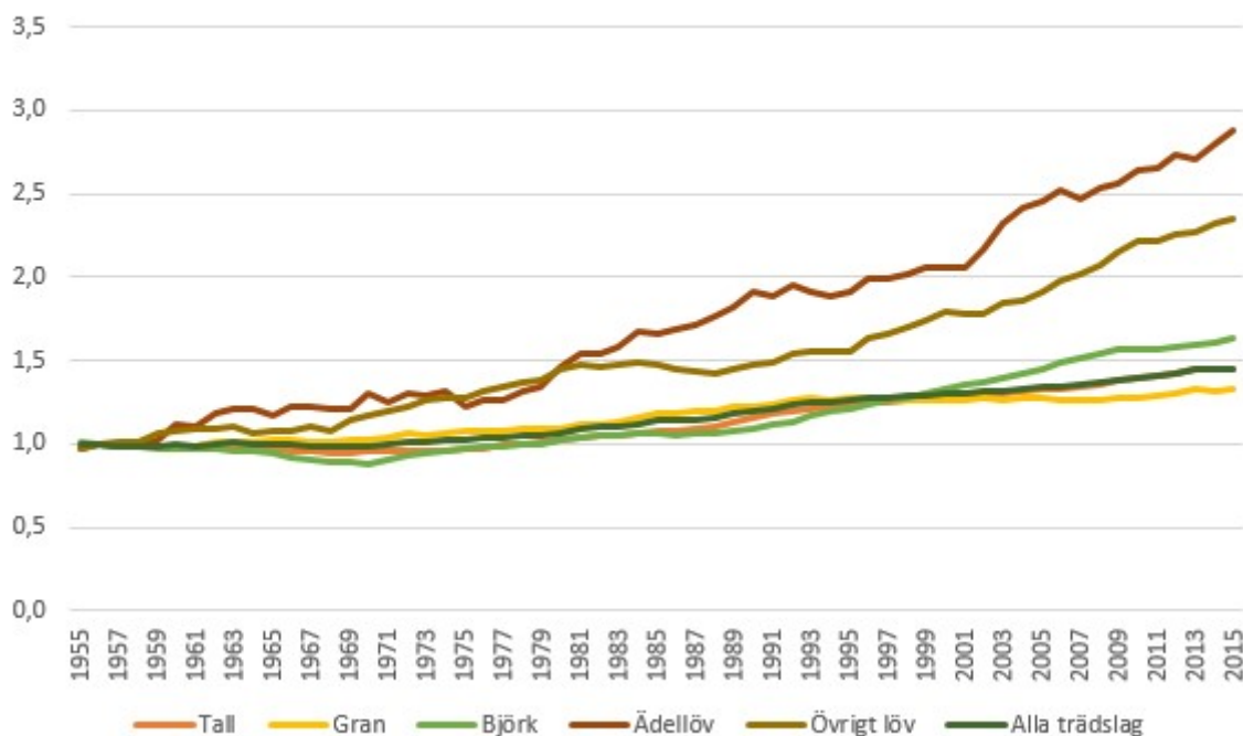
Totalt virkesförråd i Sverige av respektive trädslag. Relativ förändring 1955 = 1, underlag från Rikstaxen
